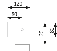
Trapezplatte 12 120 x 120 cm inkl. Stützfuß Arbeitshöhe: 68–85 cm
