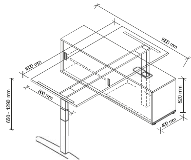
Beispiel: Tisch VXBHM 160 x 80 cm, Sidoard links montiert.
