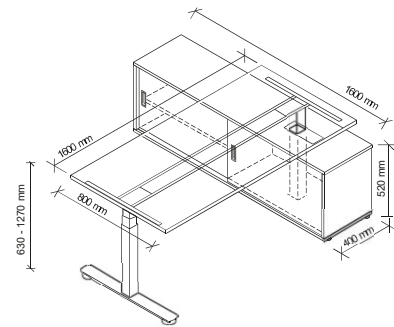
Beispiel: Tisch VXDSM 160 x 80 cm, Sidoard links montiert.
