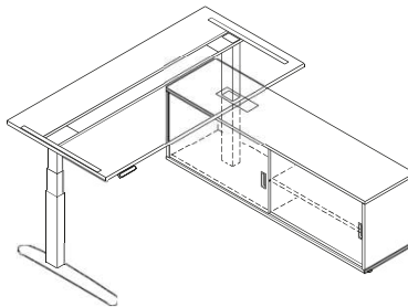
Beispiel: Tisch VXBE 160 x 80 cm, Sidoard rechts montiert.
